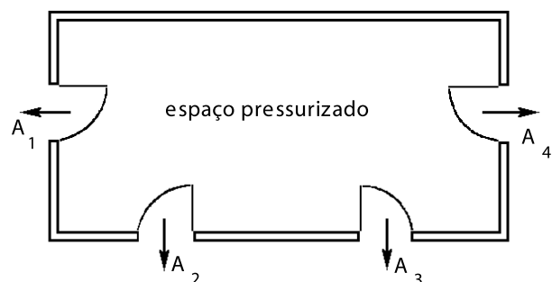
Figura 1 - Trajetórias de escape do ar em paralelo
